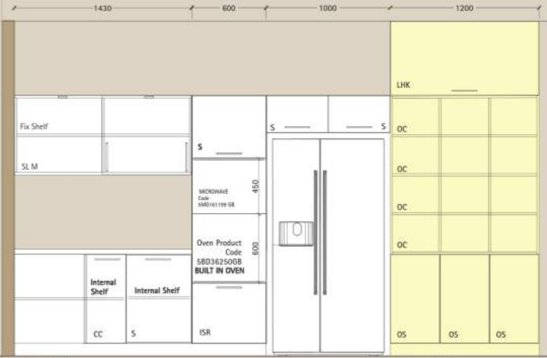
Elevation B
