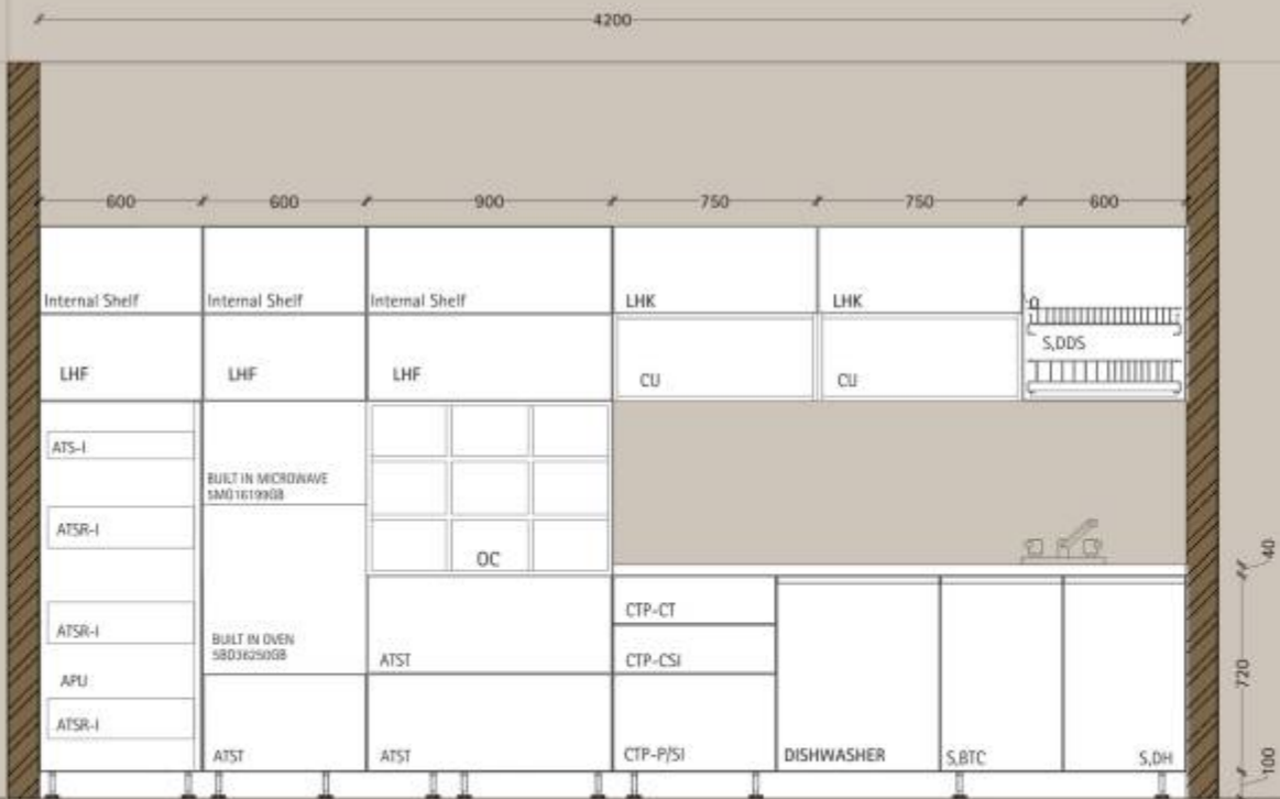
Elevation A
