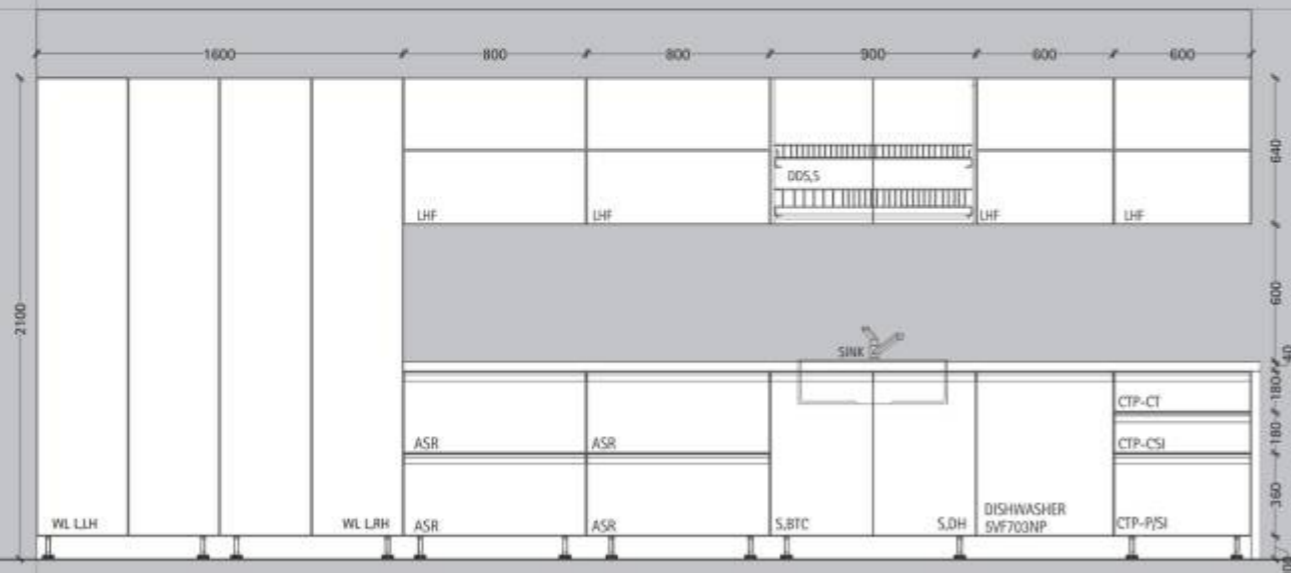
Elevation A
