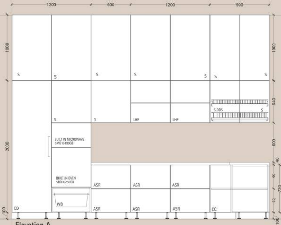
Elevation A
