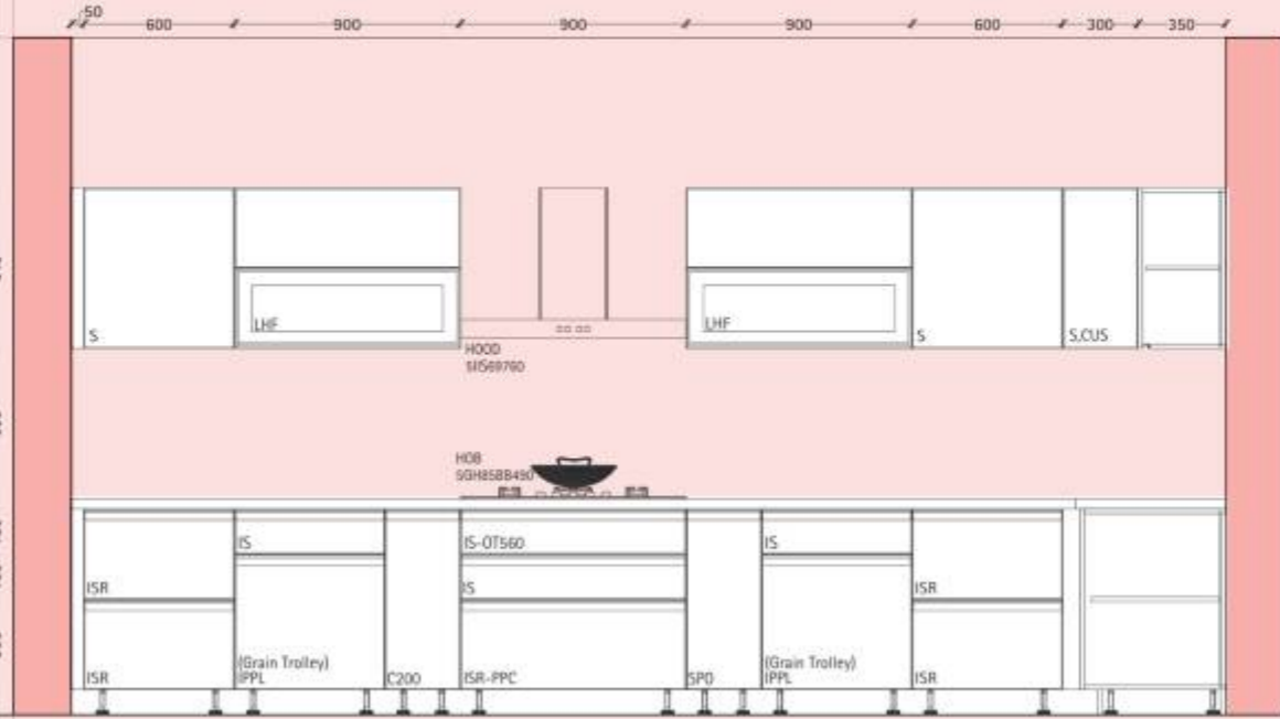
Elevation A
