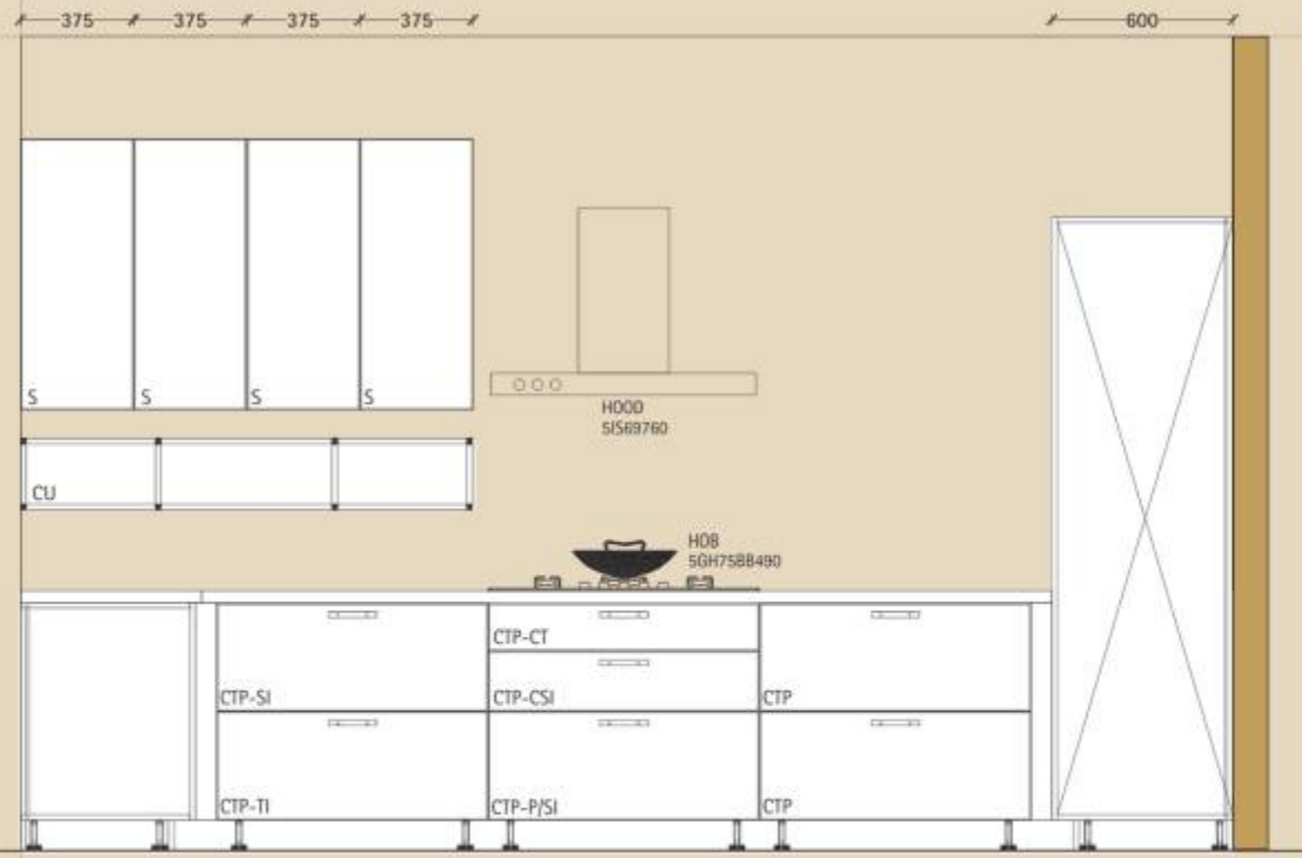
Elevation A
