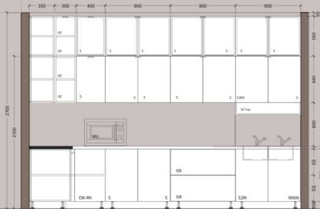
Elevation A
