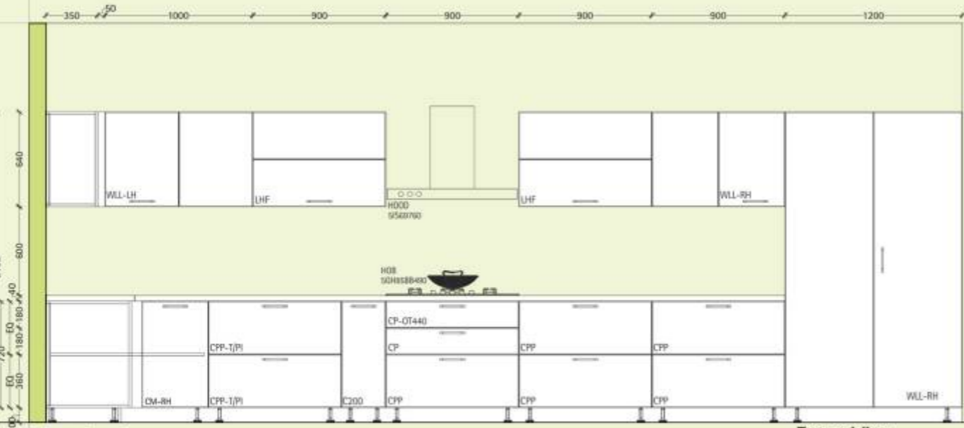
Elevation A
