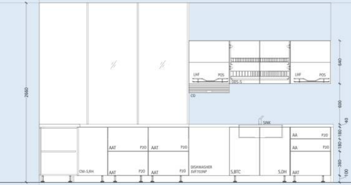
Elevation A
