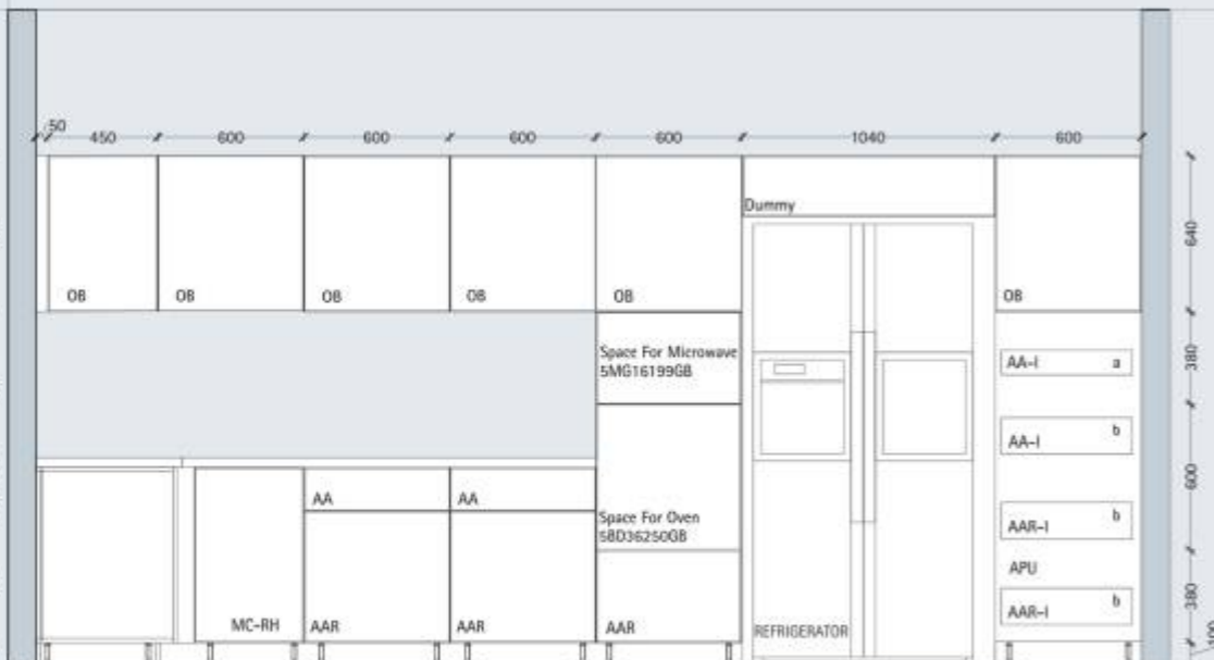
Elevation A
