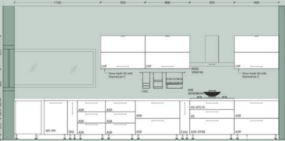
Elevation A
